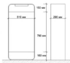
схема урны
