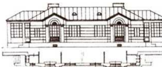
Проект деревянного дома на две квартиры в Кратовском поселке
